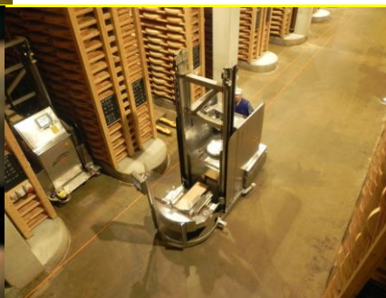
Ligne robotisée
