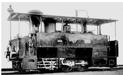
La première locomotive à vapeur du tramway de Valenciennes, Capots levés
